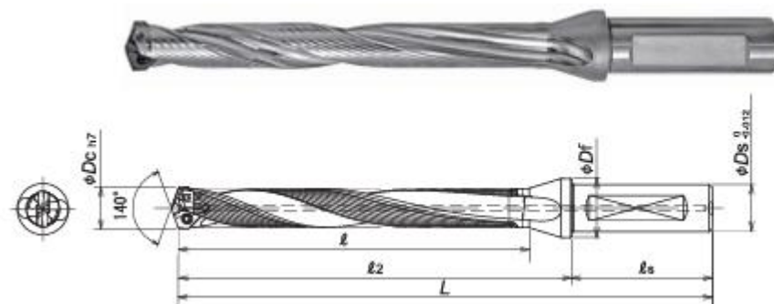
TEZDF-XL type (L/D=8)
