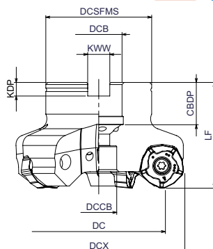
Fig. 1 \phi D_c \leq 125\text{mm}
